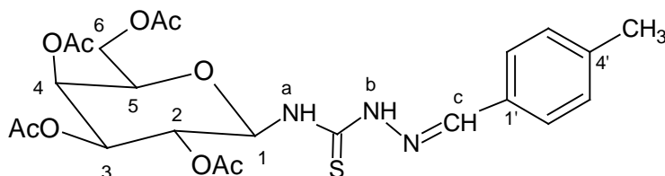
Bảng 2. Các dữ kiện phổ hồng ngoại, cộng hưởng từ hạt nhân ^1\text{H} - và ^{13}\text{C} -NMR của N-(4-methylbenzyliden)-(2,3,4,6-tetra-O- \beta -D-galactopyranosyl)thiosemicabazon
