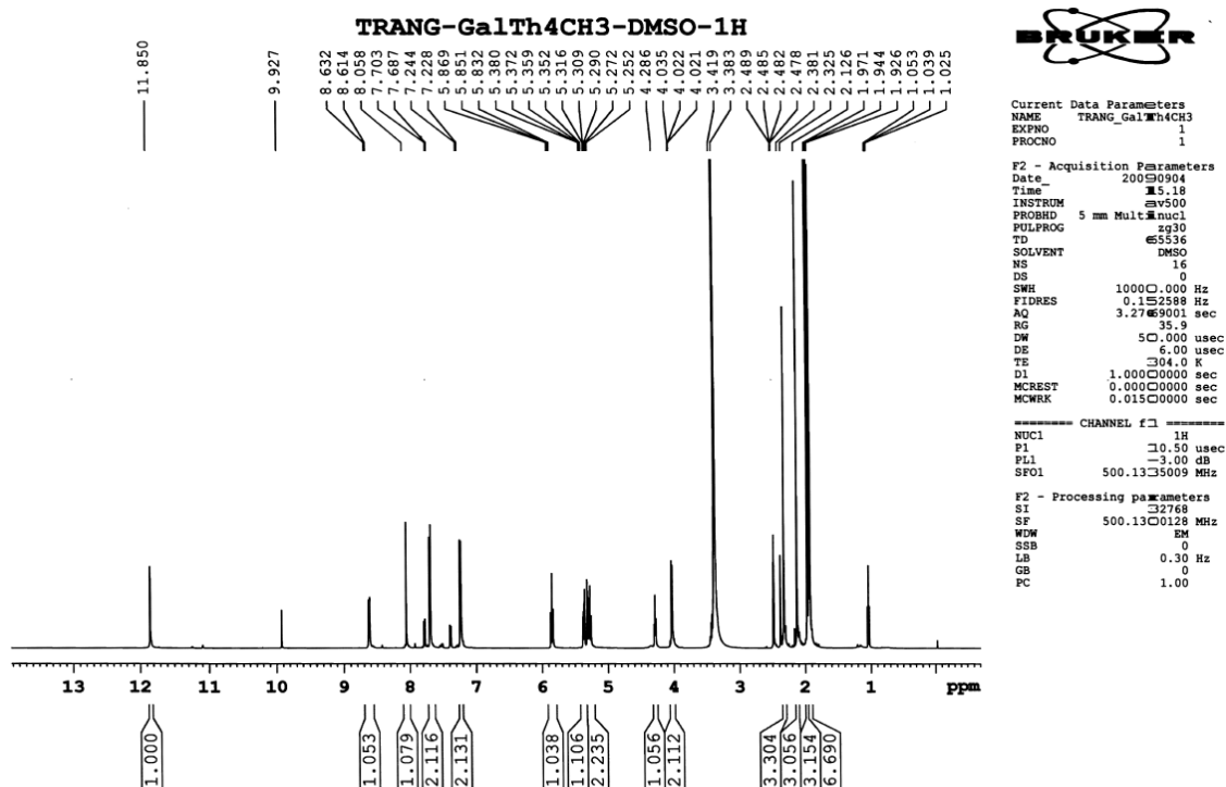
Hình 2. Phổ cộng hưởng từ hạt nhân ^1\text{H} của N-(4-metylbenzyliden)-(2,3,4,6-tetra-O- \beta -D-galactopyranozyl)thiosemicabazon
